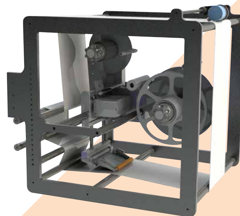
Étiqueteuse à intégrer dans une machine à forme, à remplissage et à fermeture ou dans une machine d'emballage
